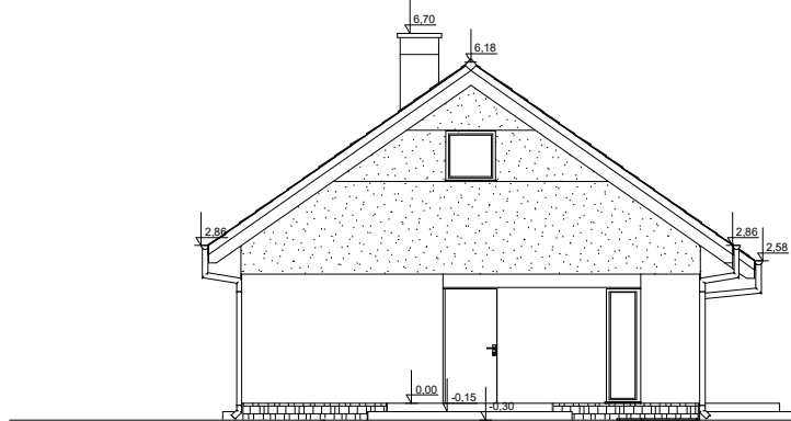
ELEWACJA FRONTOWA
