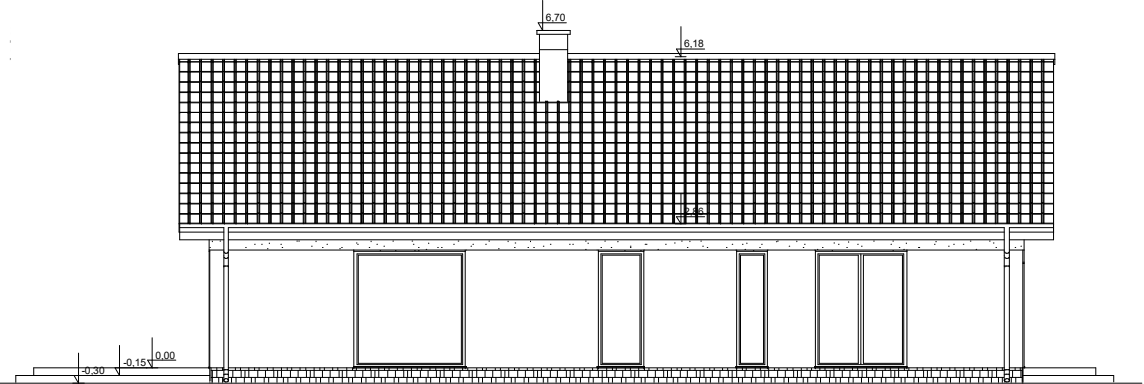
ELEWACJA BOK 1
