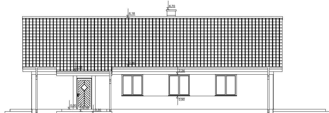
ELEWACJA BOK 2
