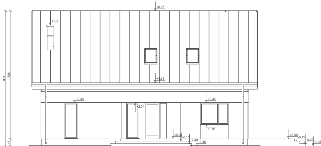
ELEWACJA FRONTOWA
