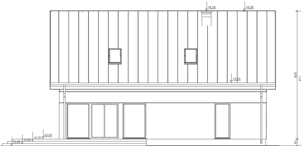
ELEWACJA OGRODOWA
