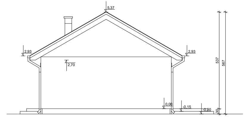
ELEWACJA BOK 2
