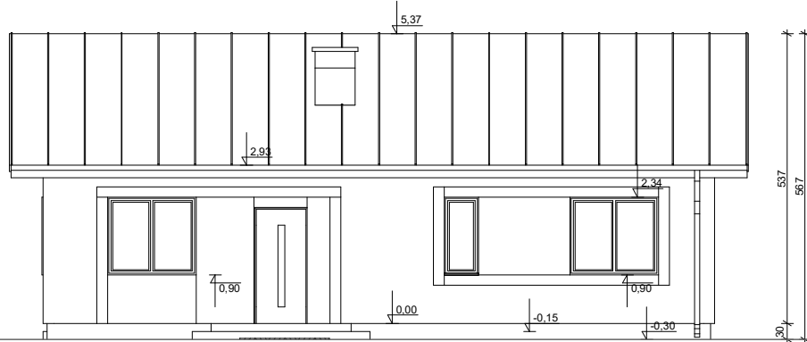
ELEWACJA FRONTOWA
