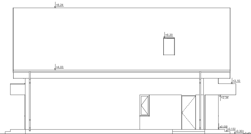
ELEWACJA BOK 1
