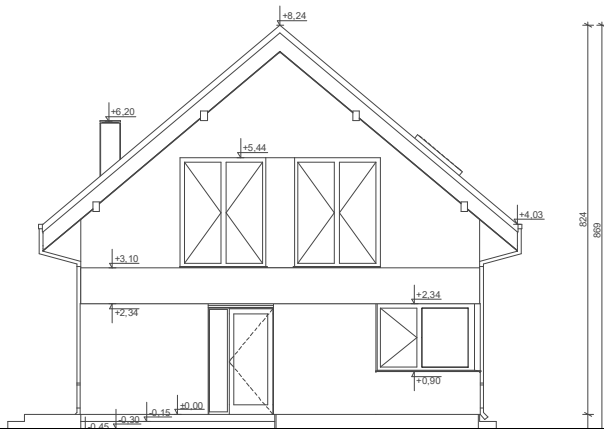
ELEWACJA FRONTOWA
