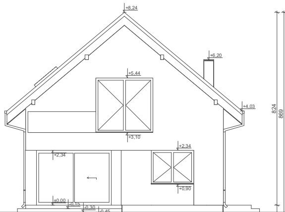
ELEWACJA TYLNA
