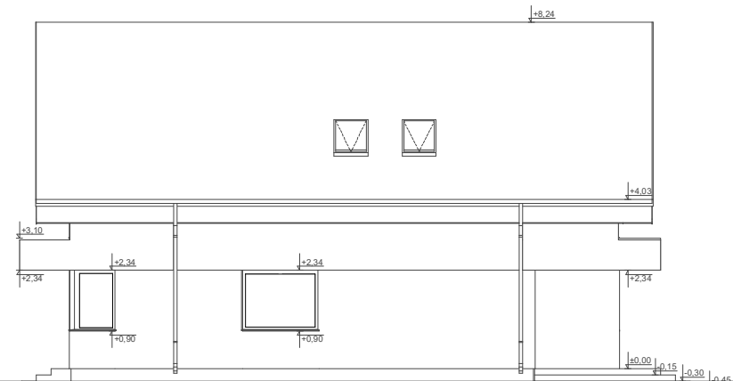
ELEWACJA BOK 2
