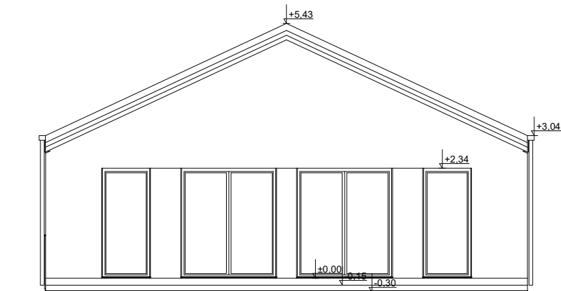
ELEWACJA OGRODOWA
