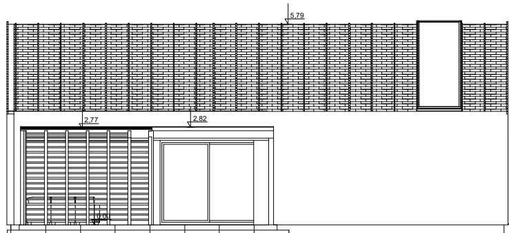
ELEWACJA ZACHODNIA
