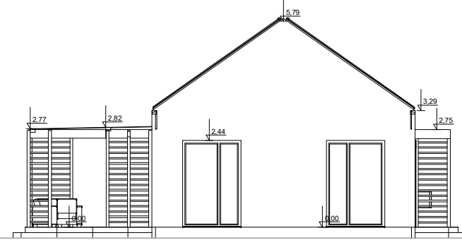
ELEWACJA POŁUDNIOWA
