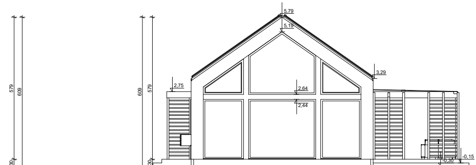
ELEWACJA PÓŁNOCNA
