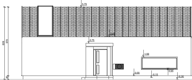
ELEWACJA WSCHODNIA
