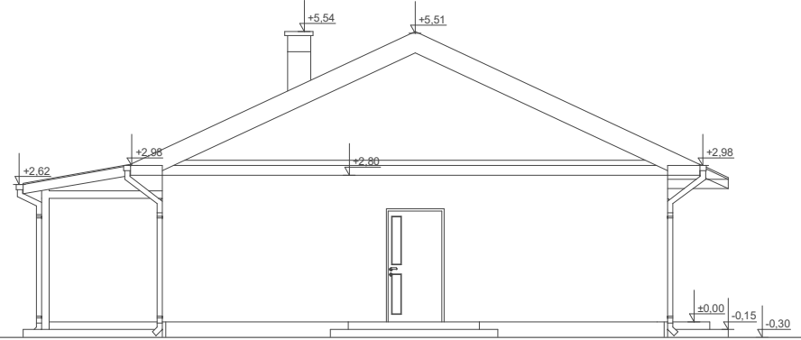
ELEWACJA BOK 1
