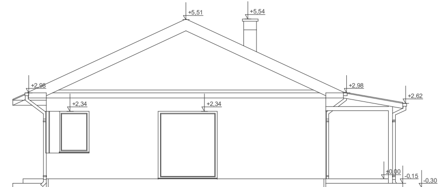
ELEWACJA BOK 2
