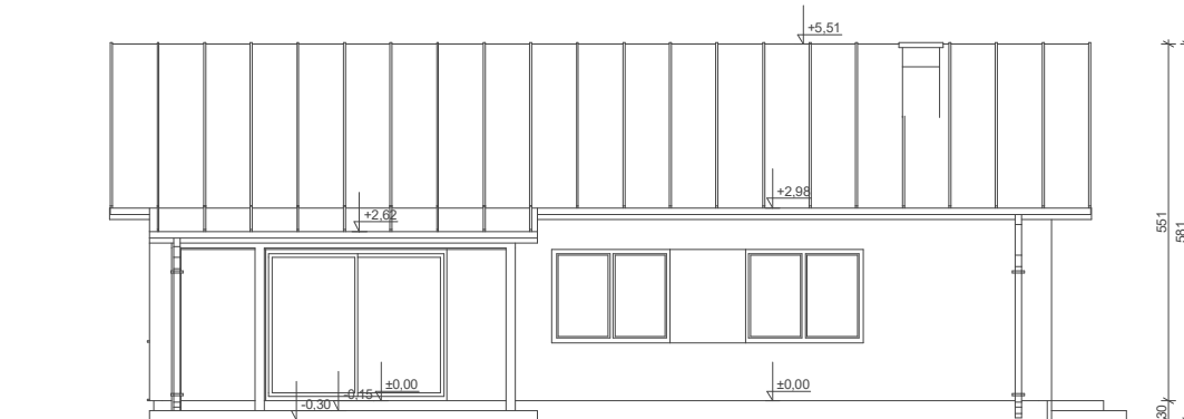
ELEWACJA OGRODOWA
