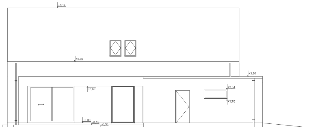
ELEWACJA BOK 2
