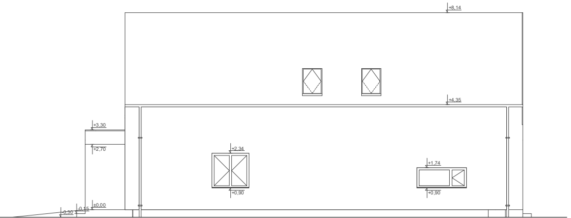
ELEWACJA BOK 1
