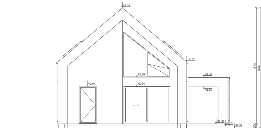
ELEWACJA OGRODOWA
