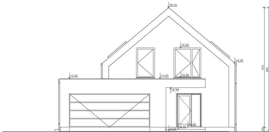
ELEWACJA FRONTOWA
