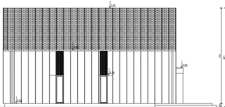
ELEWACJA ZACHODNIA
