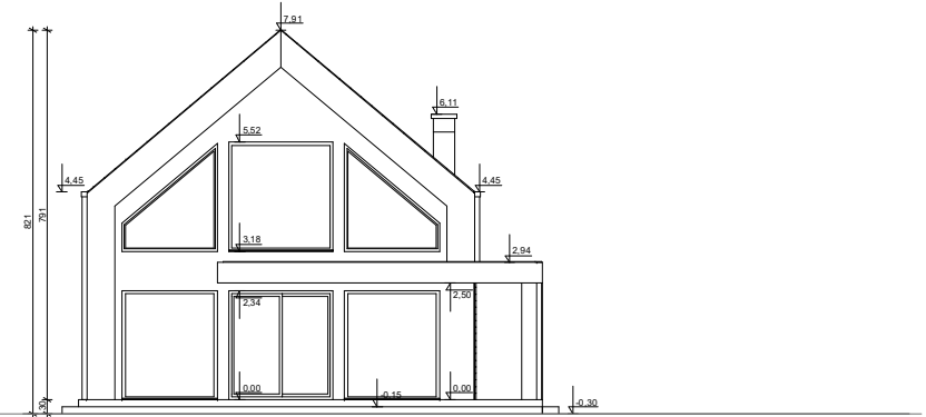
ELEWACJA POŁUDNIOWA
