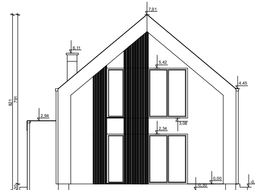
ELEWACJA PÓŁNOCNA
