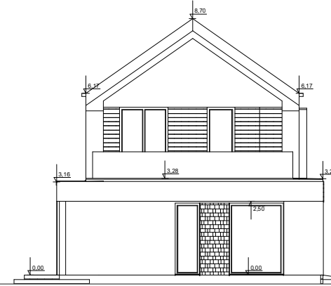
ELEWACJA ZACHODNIA
