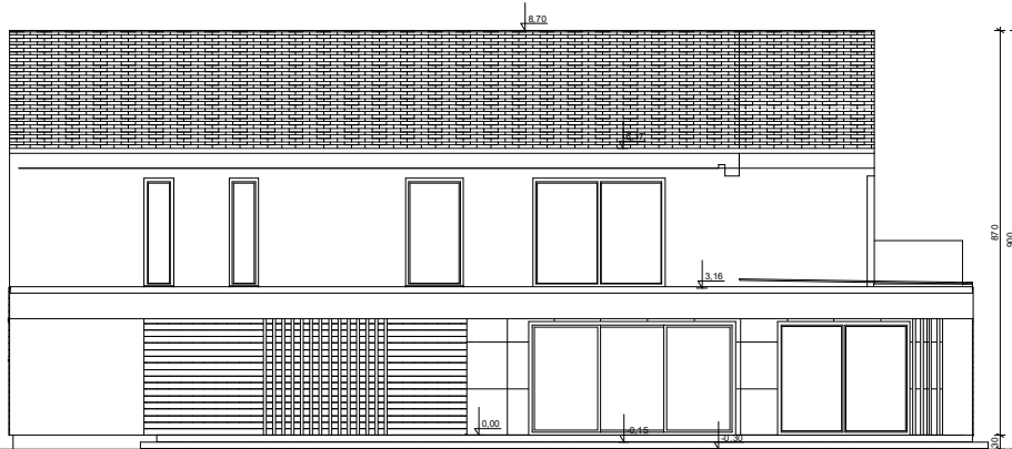
ELEWACJA PÓŁNOCNA
