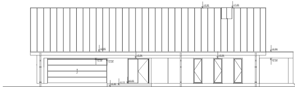
ELEWACJA FRONTOWA
