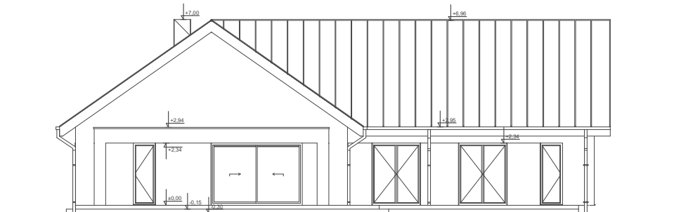
ELEWACJA BOK 2
