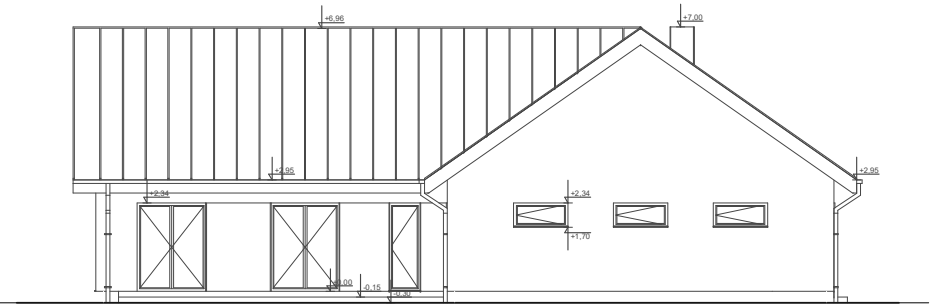
ELEWACJA BOK 1
