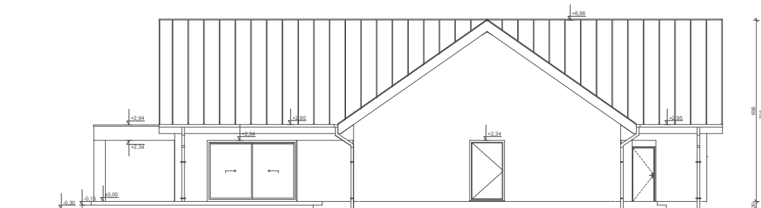
ELEWACJA OGRODOWA
