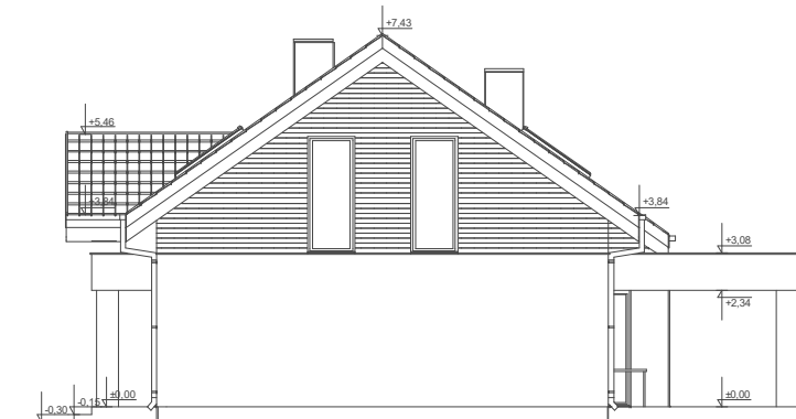
ELEWACJA BOK 2
