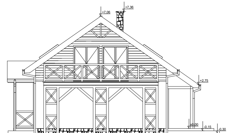
ELEWACJA BOK 2
