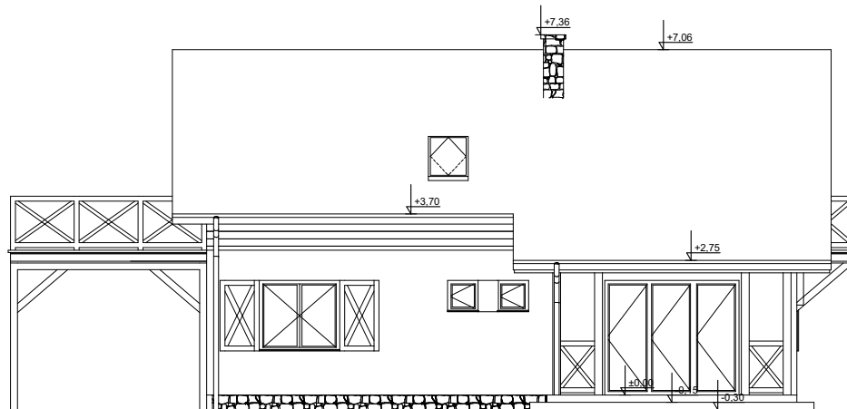
ELEWACJA OGRODOWA
