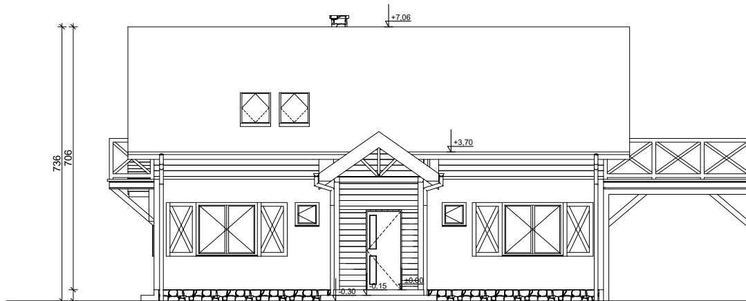
ELEWACJA FRONTOWA
