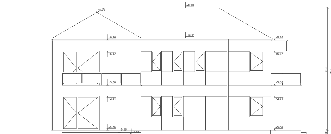
ELEWACJA OGRODOWA
