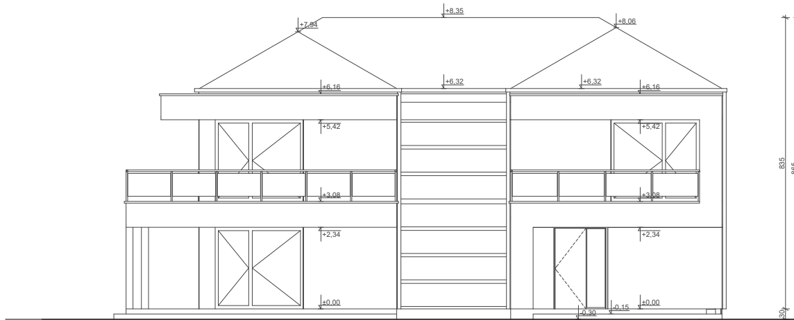
ELEWACJA FRONTOWA
