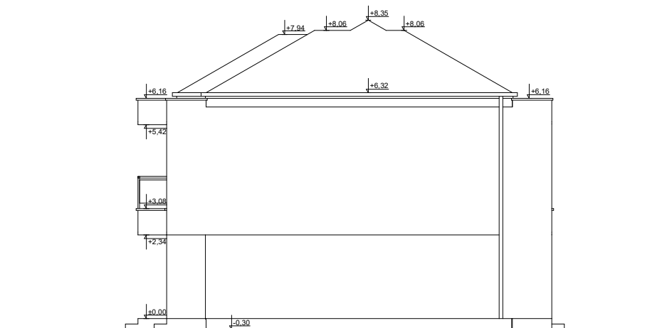
ELEWACJA BOK 2
