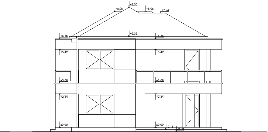
ELEWACJA BOK 1
