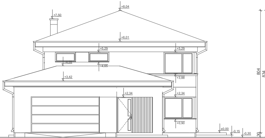
ELEWACJA FRONTOWA
