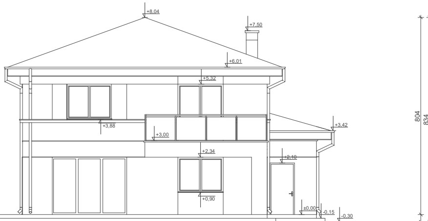
ELEWACJA OGRODOWA
