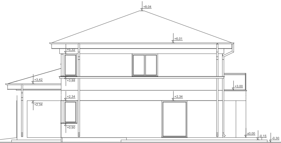
ELEWACJA BOK 1
