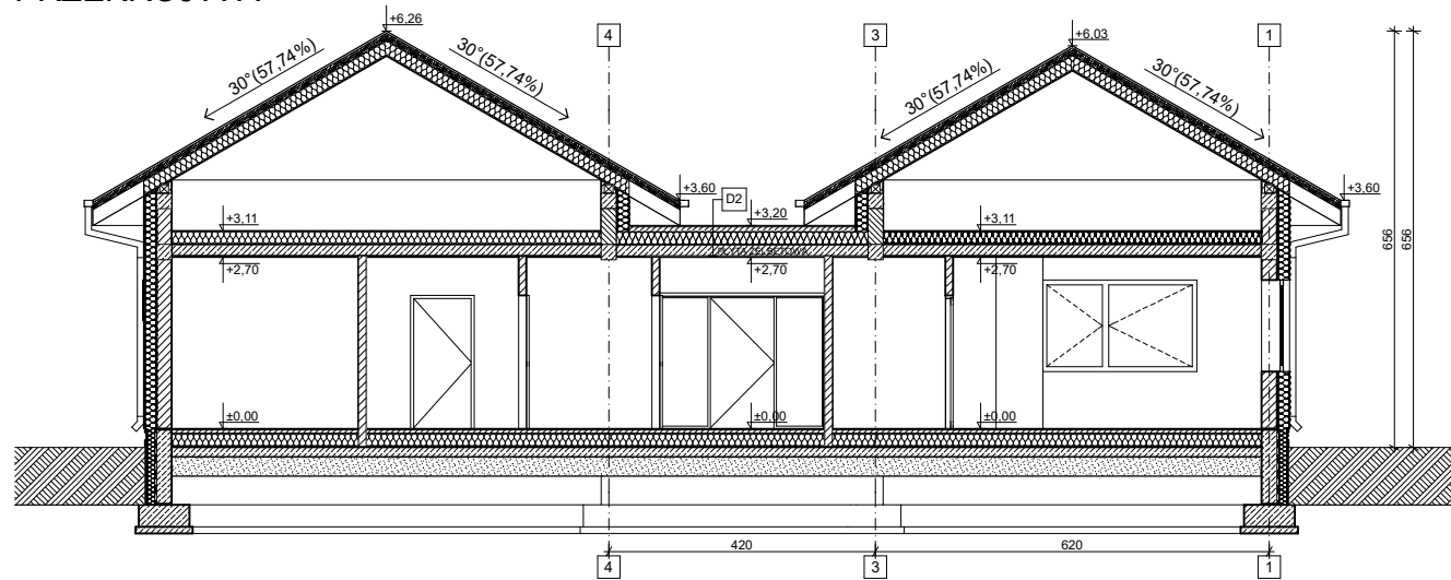
PRZEKRÓJ B-B
