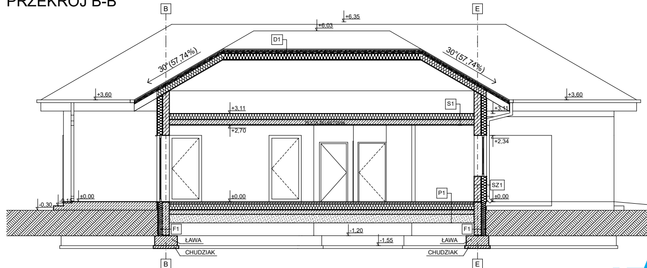
PRZEKRÓJ B-B
