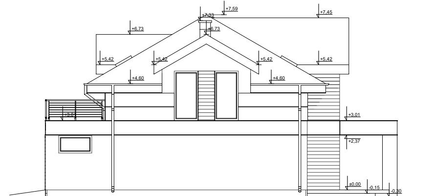
ELEWACJA BOK 2
