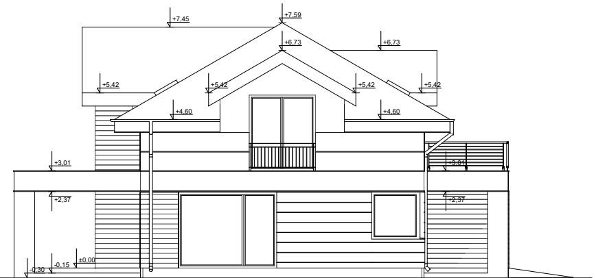
ELEWACJA BOK 1
