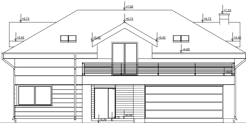
ELEWACJA FRONTOWA
