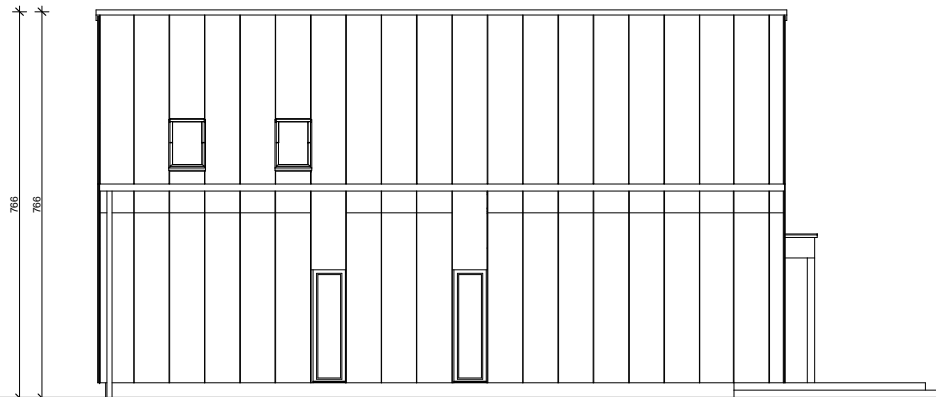
ELEWACJA OGRODOWA
