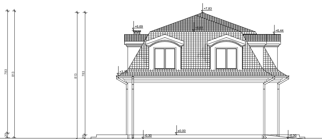
ELEWACJA BOK 1
