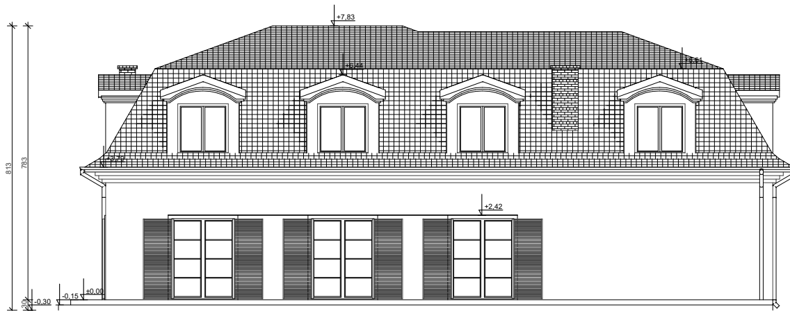
ELEWACJA OGRODOWA
