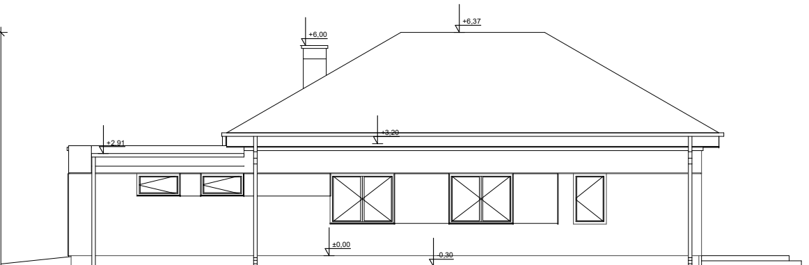
ELEWACJA BOK 2
