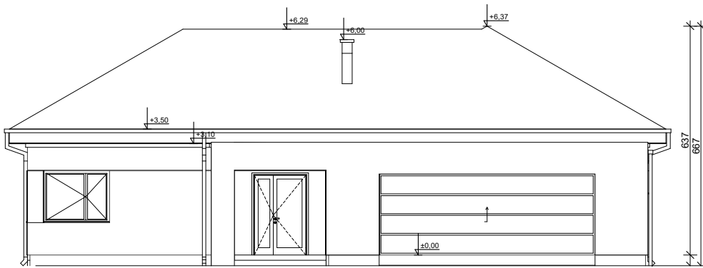
ELEWACJA FRONTOWA
