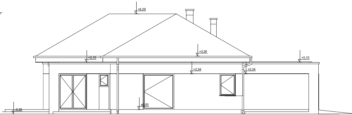
ELEWACJA BOK 1
