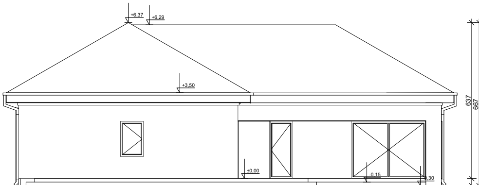
ELEWACJA OGRODOWA
