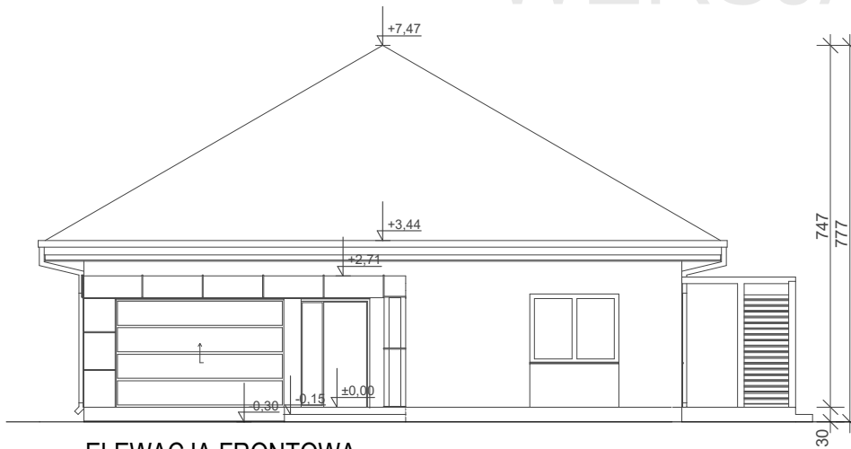
ELEWACJA FRONTOWA
