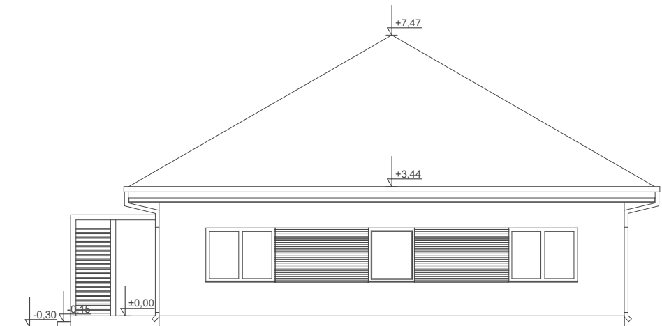
ELEWACJA OGRODOWA
