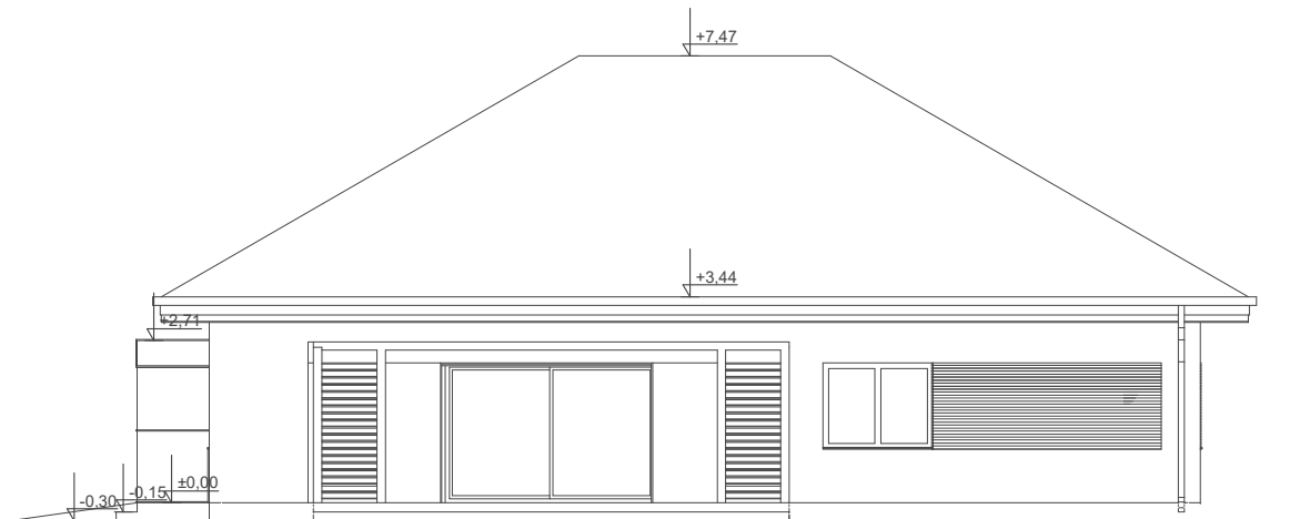
ELEWACJA BOK 2
