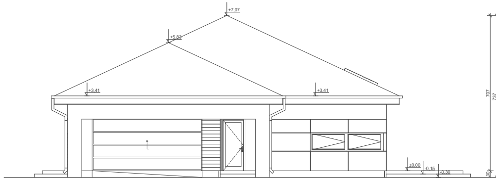
ELEWACJA FRONTOWA
