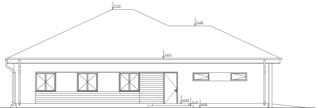
ELEWACJA BOK 1
