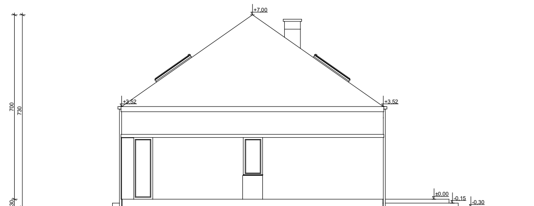
ELEWACJA BOK 2
