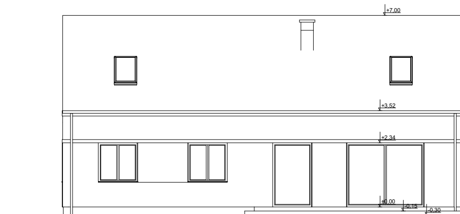
ELEWACJA OGRODOWA
