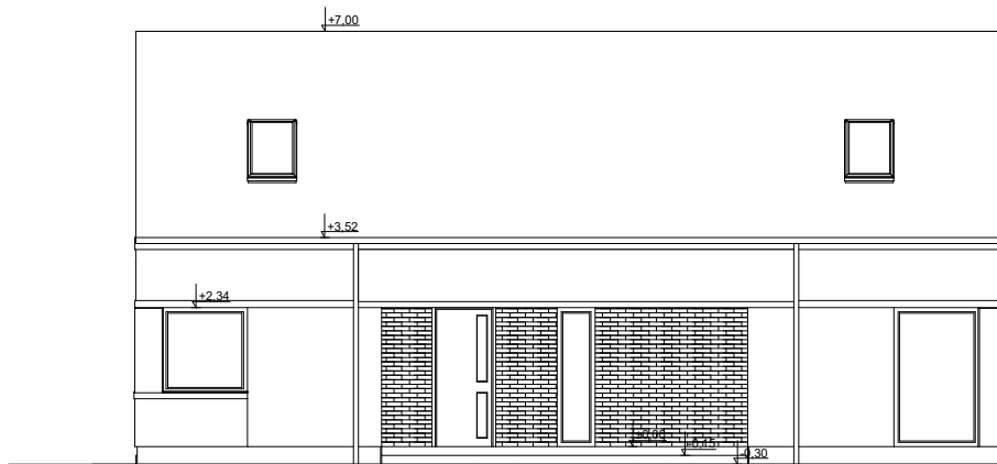
ELEWACJA FRONTOWA
