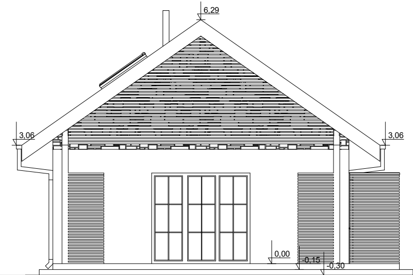
ELEWACJA OGRODOWA
