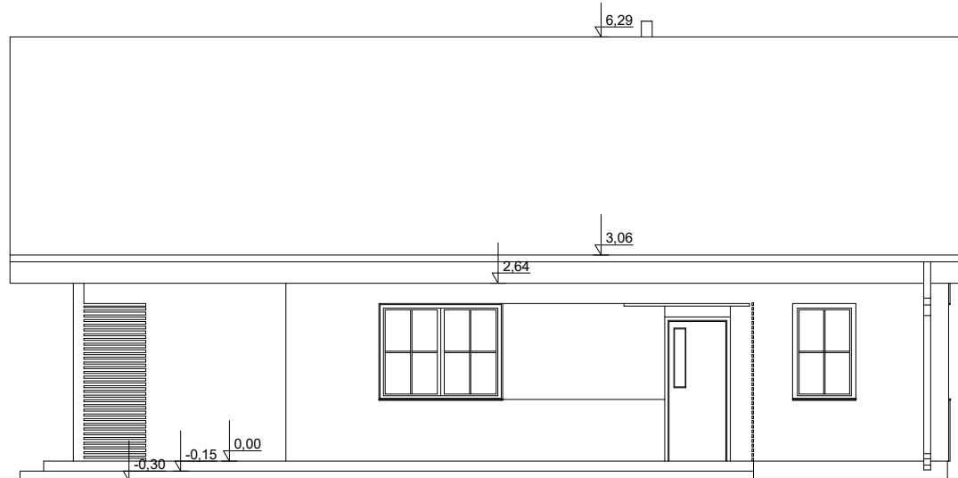
ELEWACJA FRONTOWA
