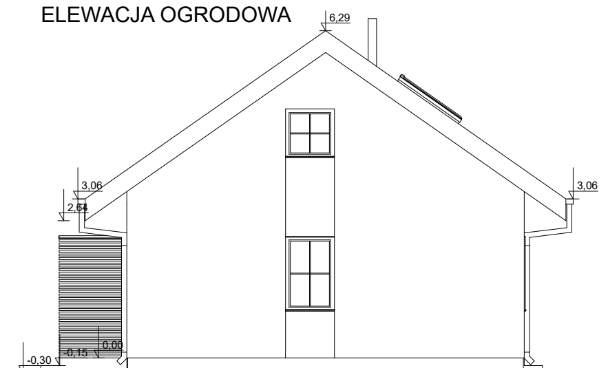
ELEWACJA BOK 2
