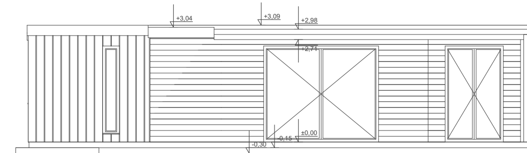
ELEWACJA FRONTOWA
