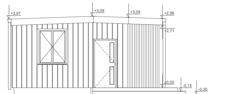
ELEWACJA BOK 2
