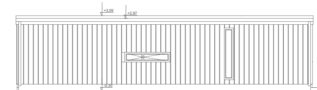
ELEWACJA OGRODOWA
