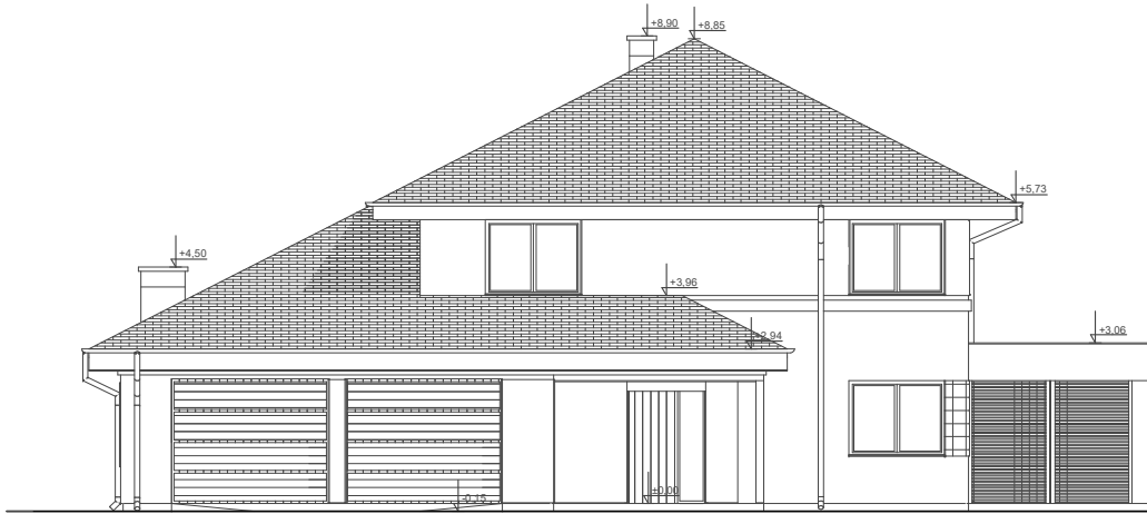
ELEWACJA FRONTOWA
