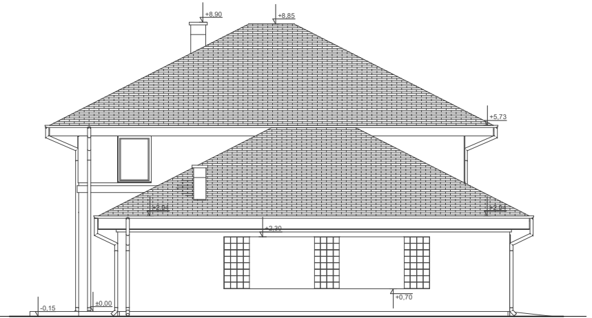
ELEWACJA BOK 1
