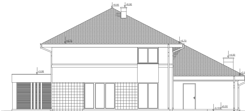
ELEWACJA OGRODOWA
