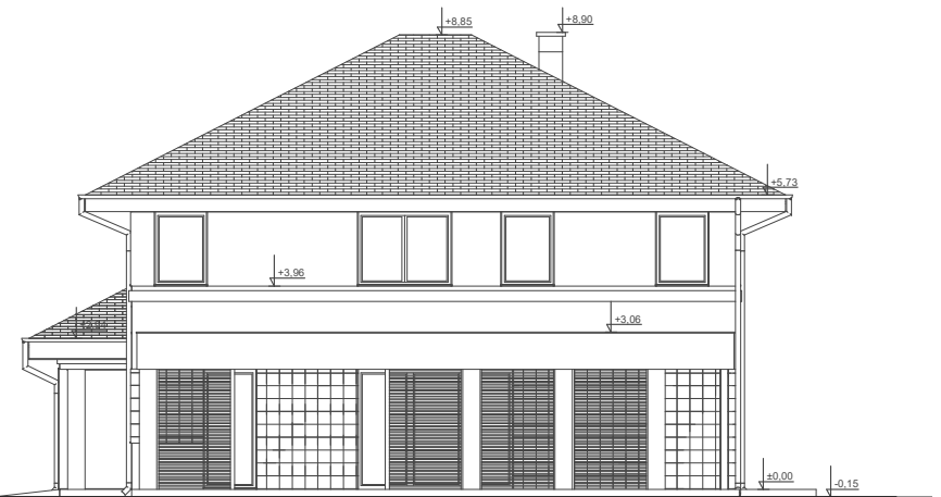
ELEWACJA BOK 2
