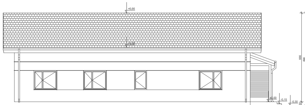
ELEWACJA OGRODOWA
