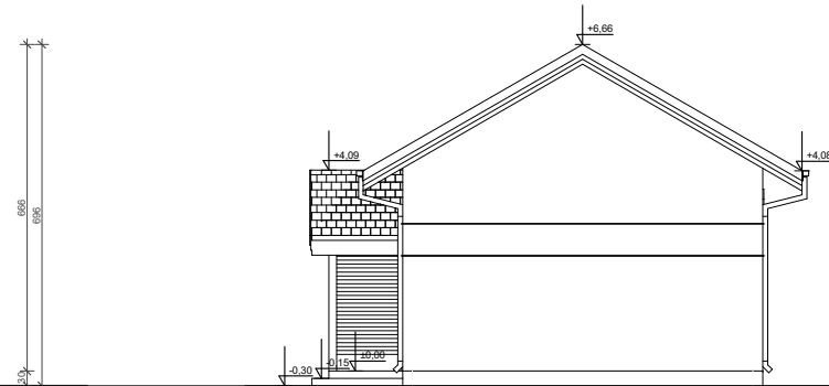
ELEWACJA BOK 1
