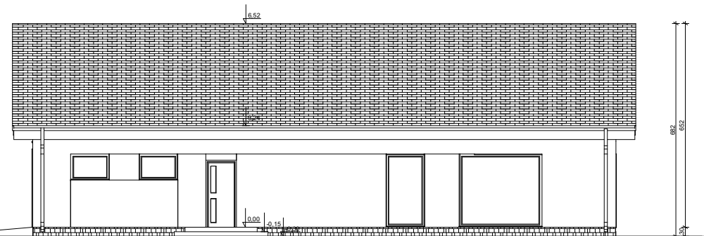
ELEWACJA BOK 2
