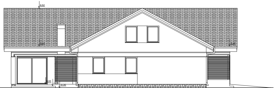
ELEWACJA BOK 1
