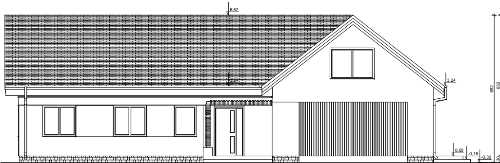
ELEWACJA FRONTOWA
