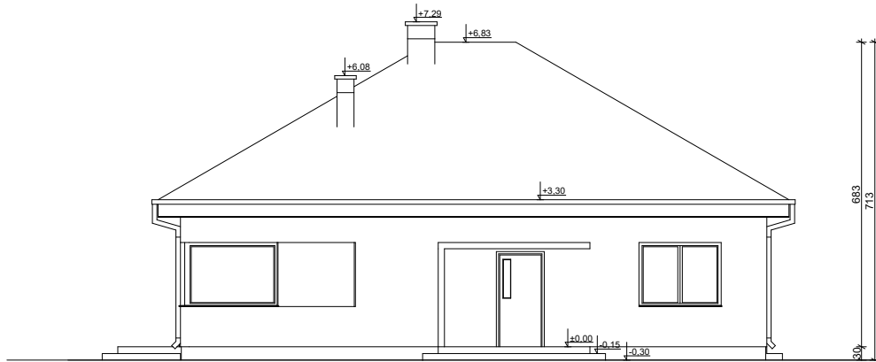
ELEWACJA FRONTOWA
