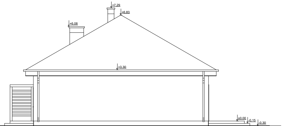
ELEWACJA BOK 2
