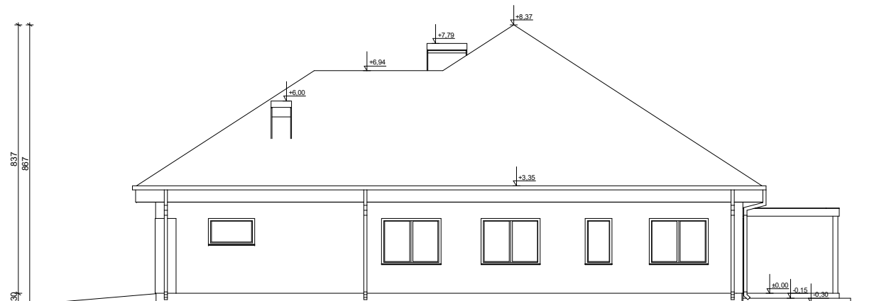
ELEWACJA BOK 2
