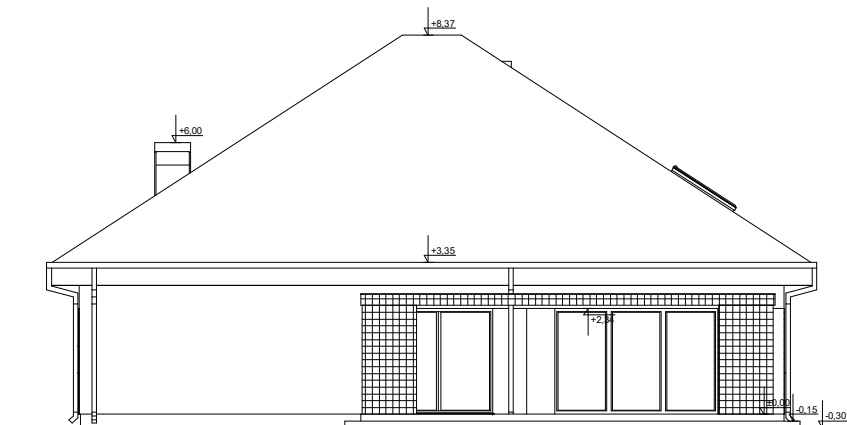
ELEWACJA OGRODOWA
