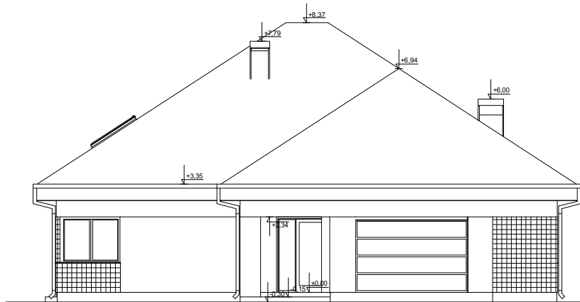
ELEWACJA FRONTOWA
