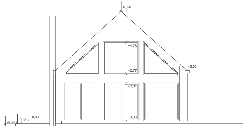
ELEWACJA BOK 2
