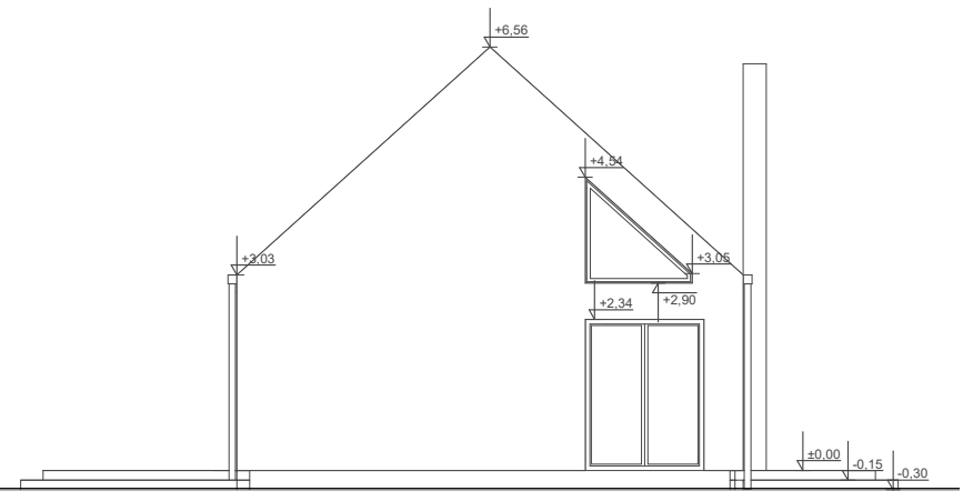
ELEWACJA BOK 1
