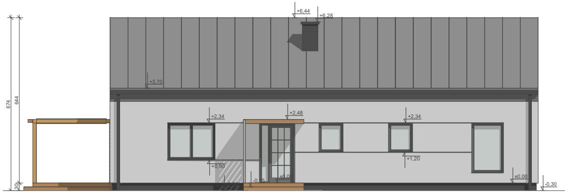
ELEWACJA FRONTOWA
