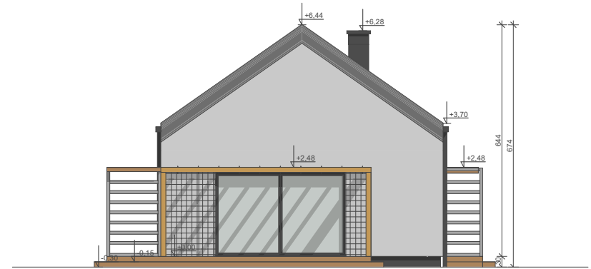
ELEWACJA BOK 1
