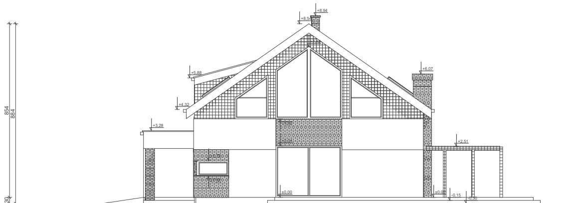
ELEWACJA BOK 2
