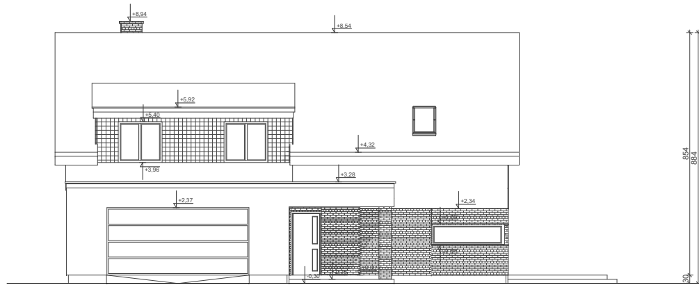
ELEWACJA FRONTOWA
