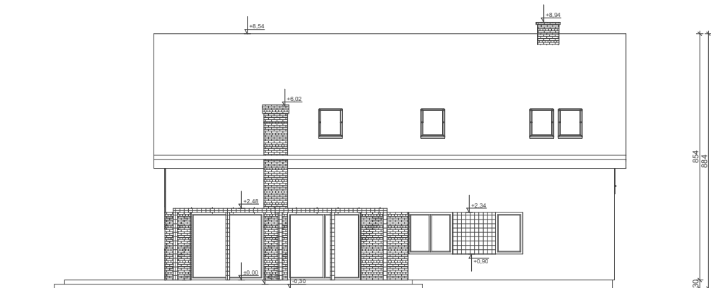
ELEWACJA OGRODOWA
