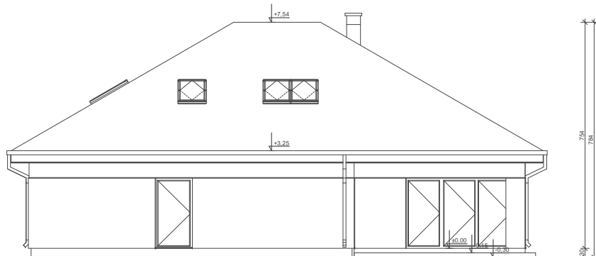
ELEWACJA OGRODOWA
