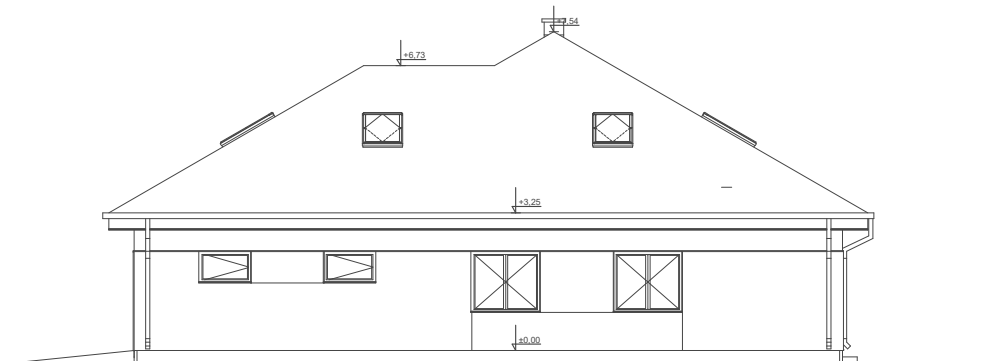
ELEWACJA BOK 2
