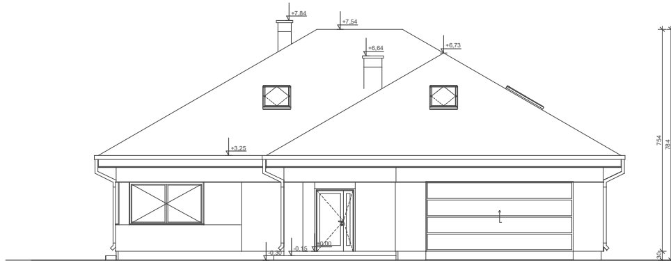
ELEWACJA FRONTOWA
