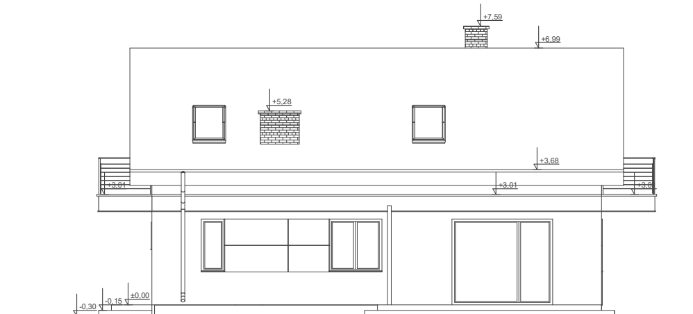
ELEWACJA OGRODOWA
