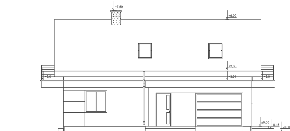
ELEWACJA FRONTOWA
