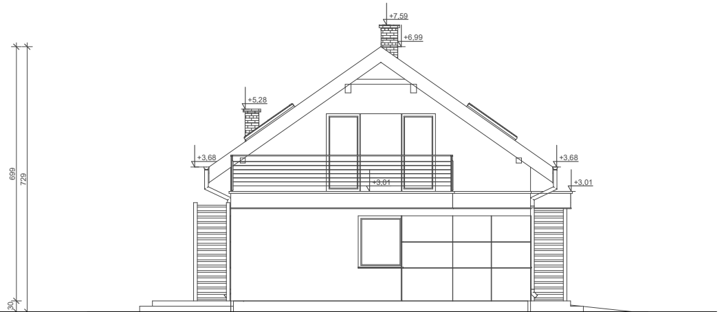
ELEWACJA BOK 1
