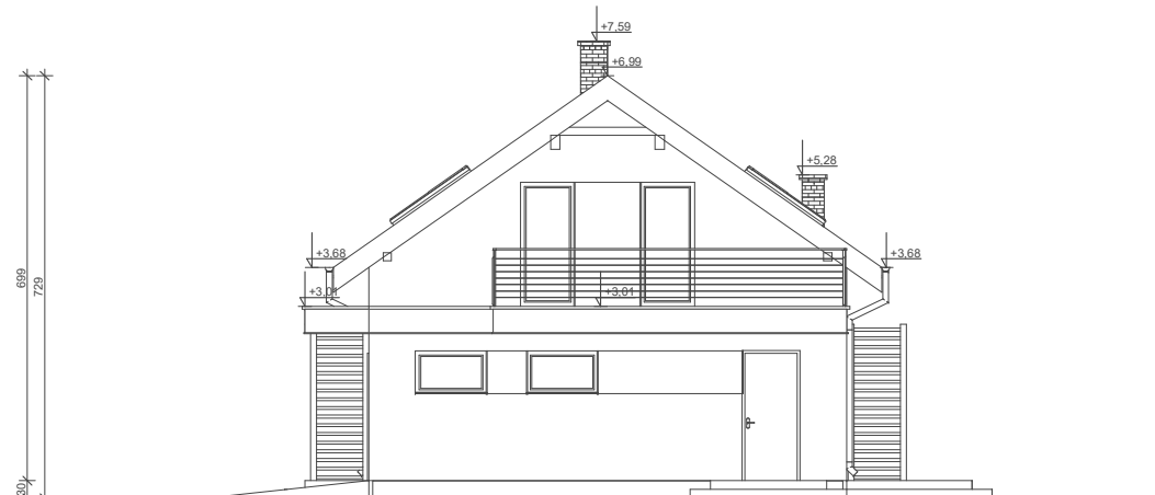
ELEWACJA BOK 2
