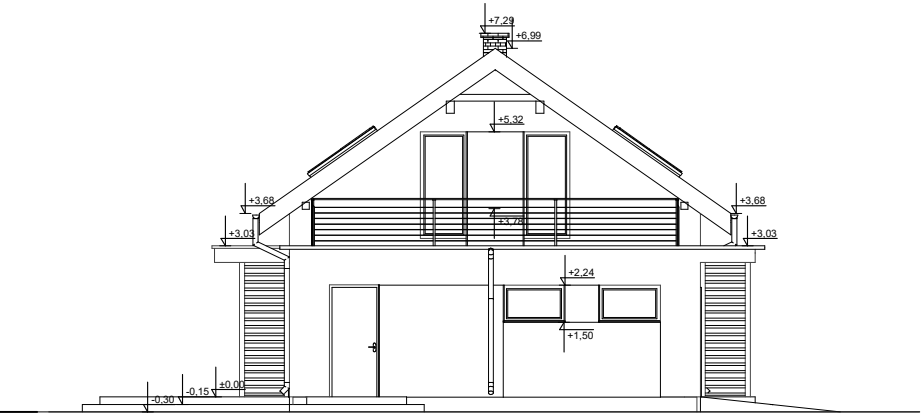
ELEWACJA BOK 1
