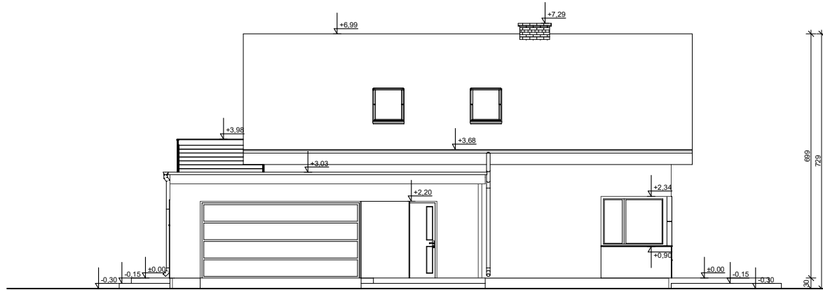
ELEWACJA FRONTOWA
