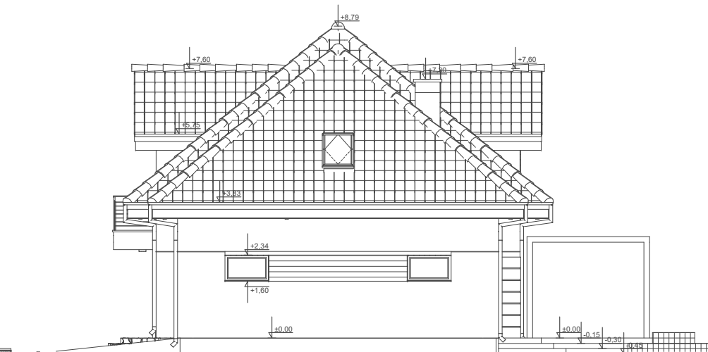
ELEWACJA BOK 2
