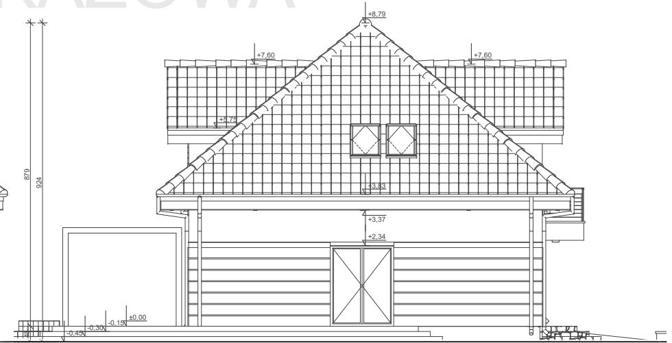
ELEWACJA BOK 1
