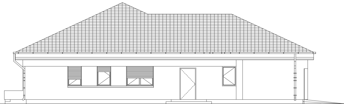
ELEWACJA BOK 2
