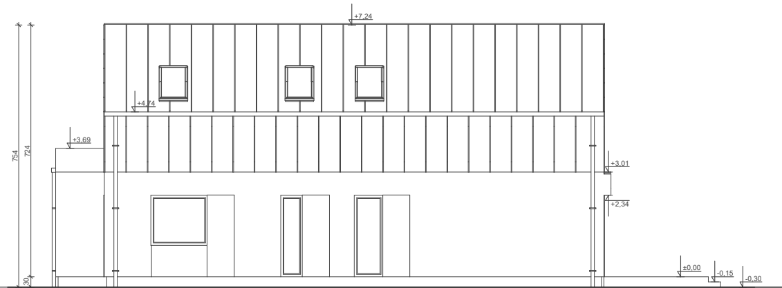
ELEWACJA BOK 1
