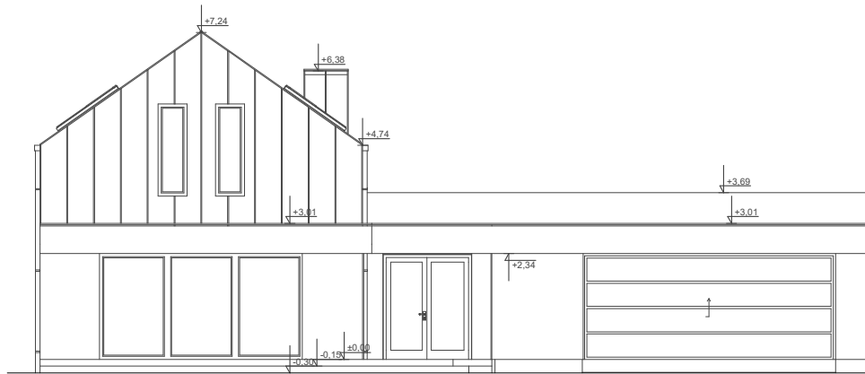
ELEWACJA FRONTOWA
