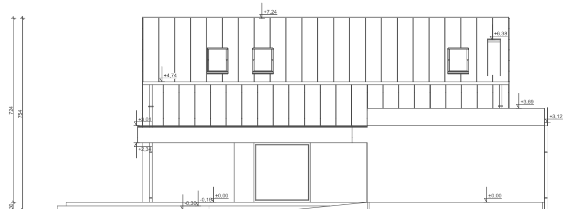
ELEWACJA BOK 2
