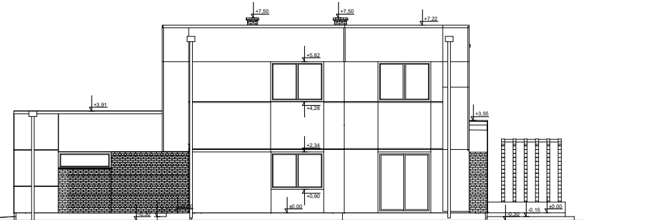
ELEWACJA BOK 2
