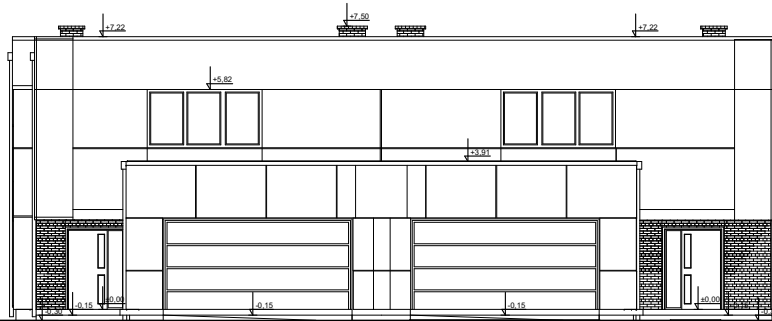
ELEWACJA FRONTOWA
