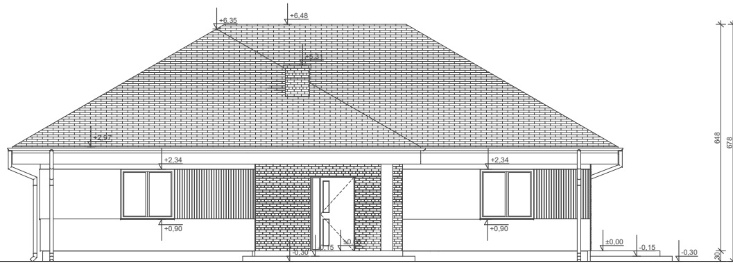
ELEWACJA FRONTOWA
