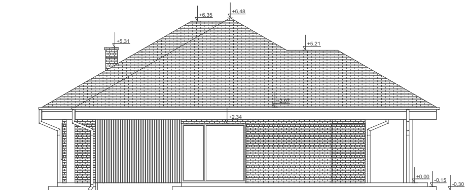
ELEWACJA BOK 2
