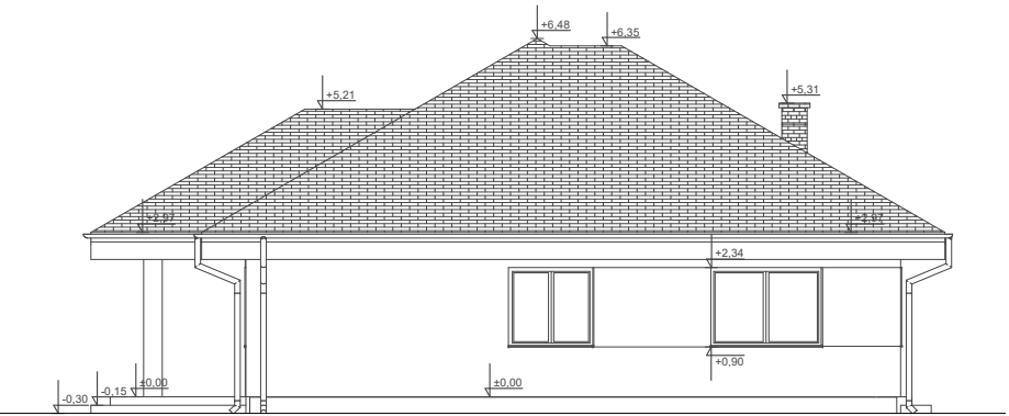
ELEWACJA BOK 1
