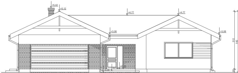
ELEWACJA FRONTOWA
