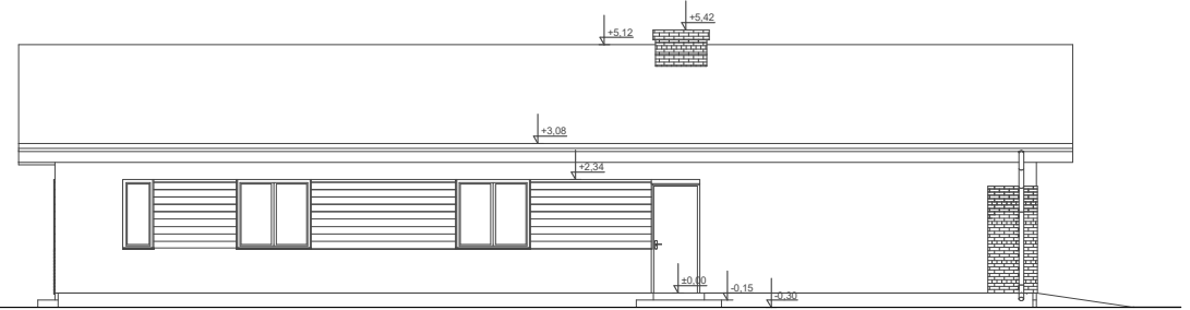
ELEWACJA BOK 1
