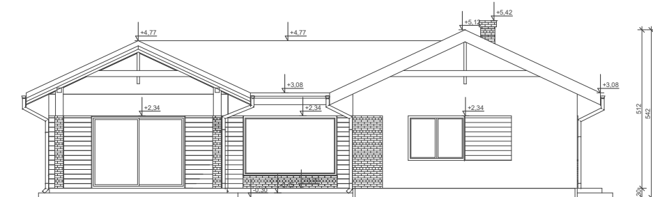
ELEWACJA OGRODOWA
