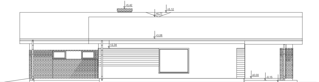
ELEWACJA BOK 2
