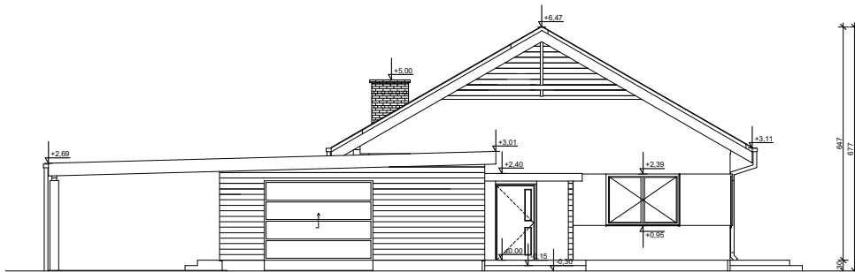
ELEWACJA FRONTOWA
