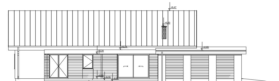
ELEWACJA BOK 2
