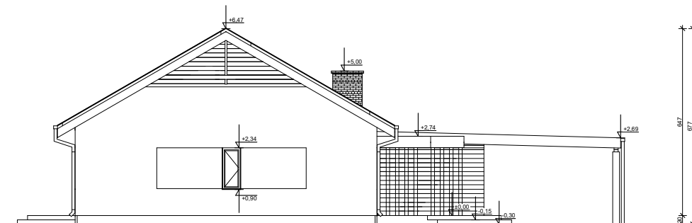
ELEWACJA OGRODOWA
