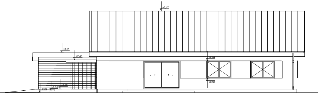
ELEWACJA BOK 1
