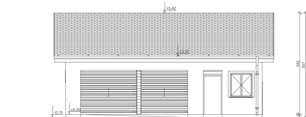
ELEWACJA FRONTOWA
