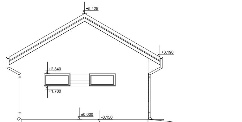
ELEWACJA BOK 1
