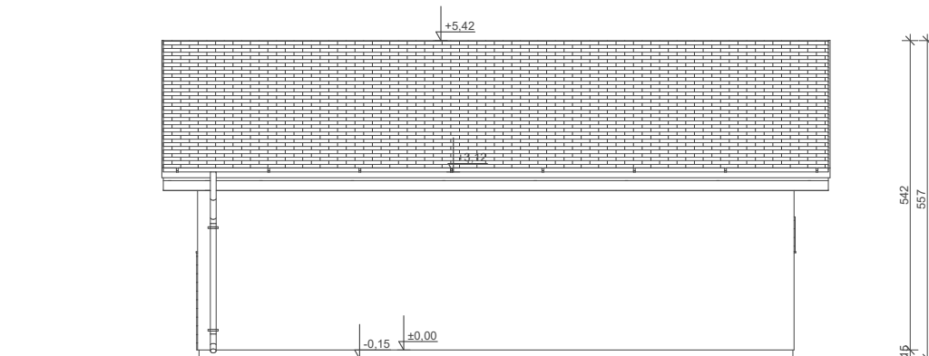
ELEWACJA OGRODOWA
