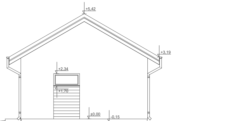
ELEWACJA BOK 2
