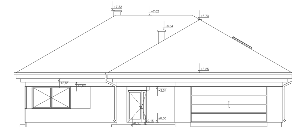
ELEWACJA FRONTOWA
