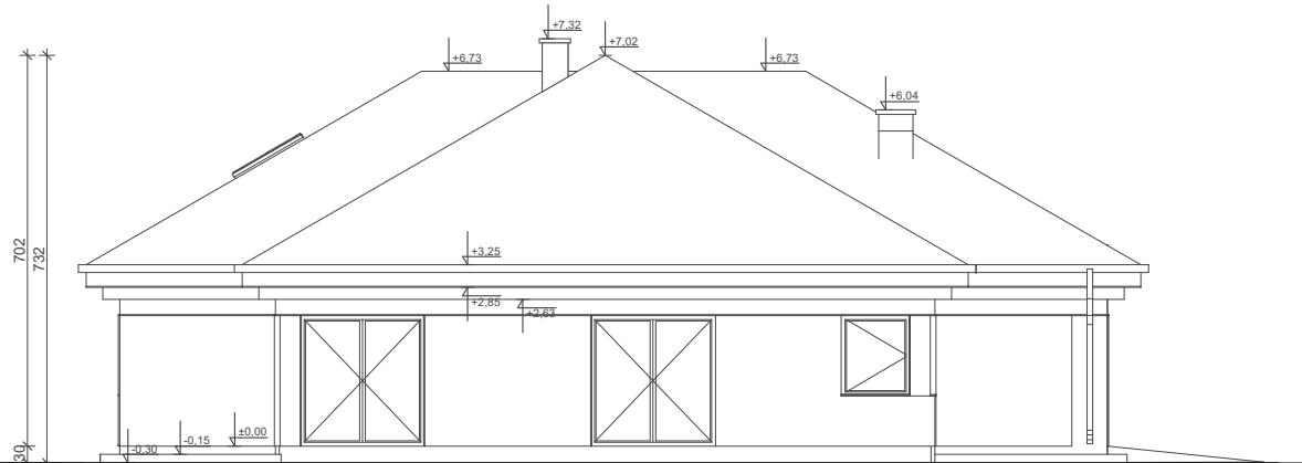
ELEWACJA BOK 1
