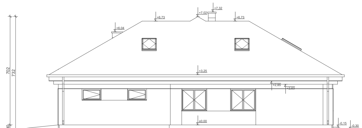
ELEWACJA BOK 2
