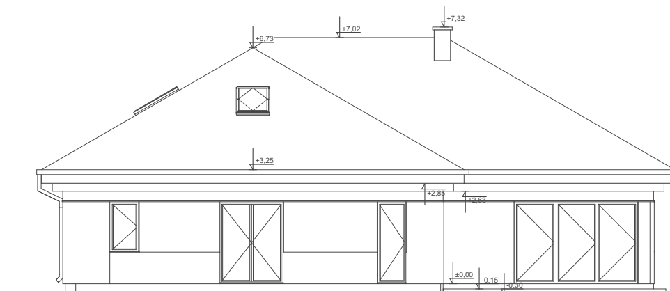
ELEWACJA OGRODOWA
