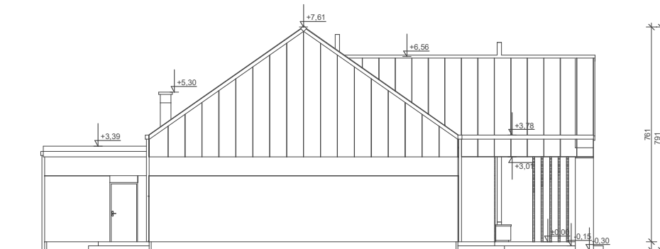
ELEWACJA OGRODOWA
