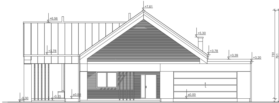
ELEWACJA FRONTOWA
