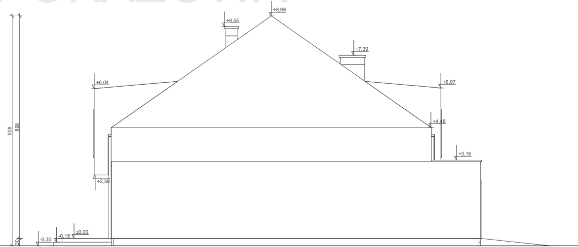
ELEWACJA BOK 1
