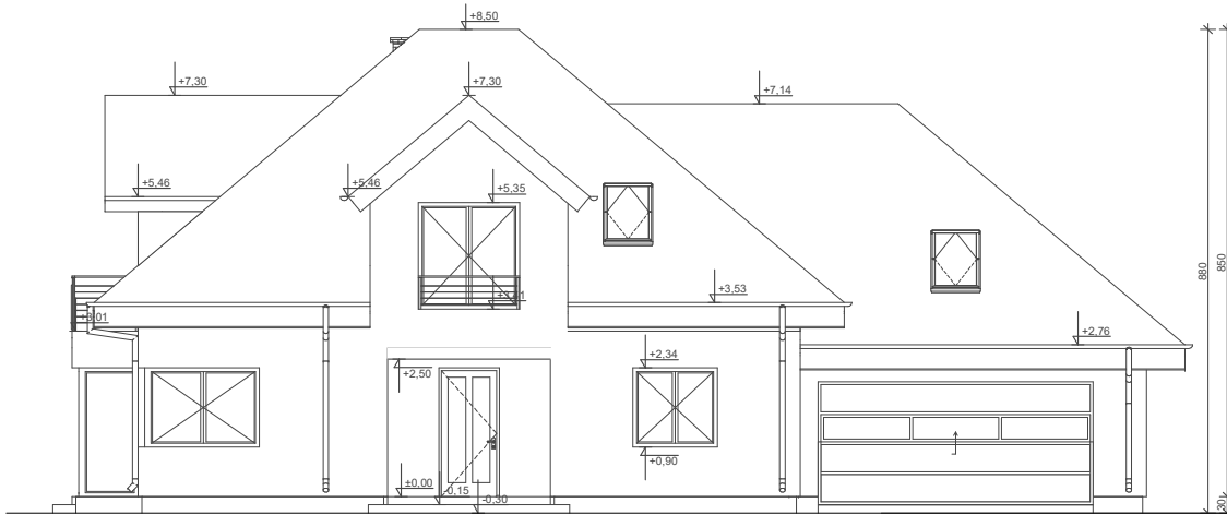
ELEWACJA FRONTOWA
