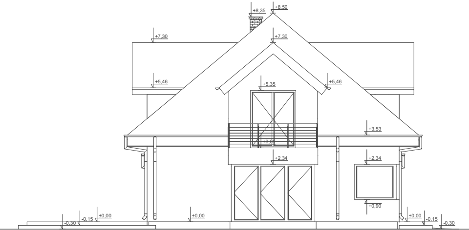
ELEWACJA BOK 1
