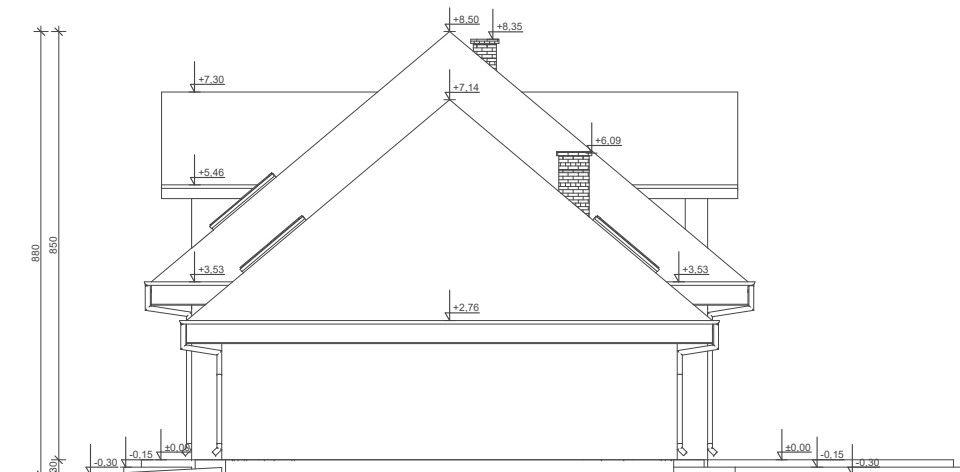
ELEWACJA BOK 2
