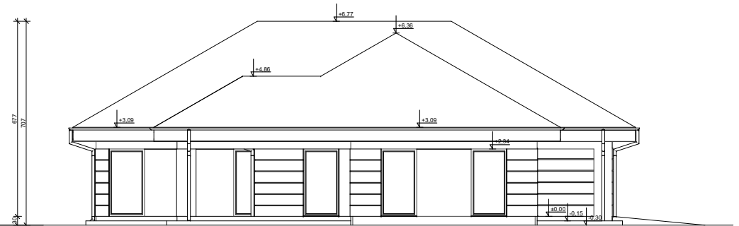
ELEWACJA BOK 1
