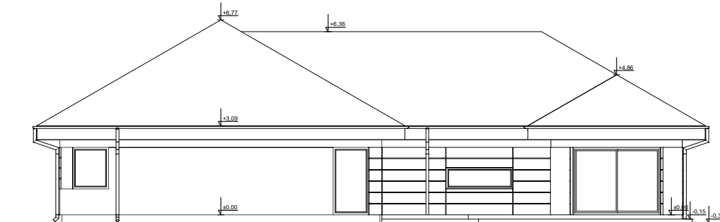
ELEWACJA OGRODOWA
