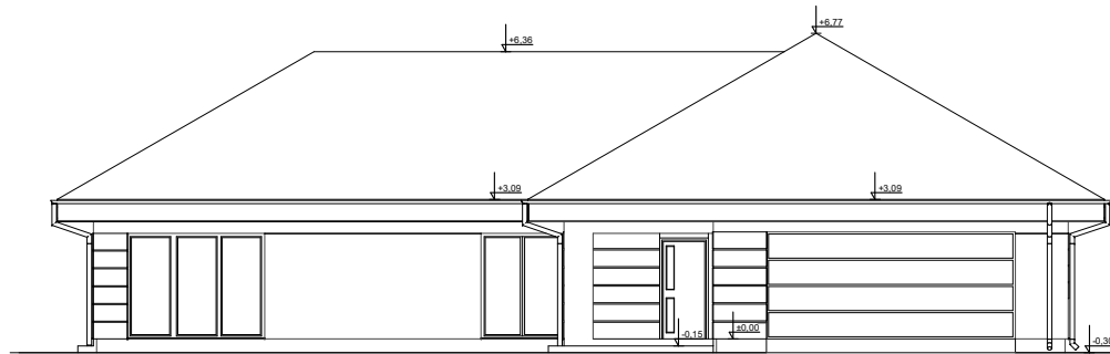
ELEWACJA FRONTOWA
