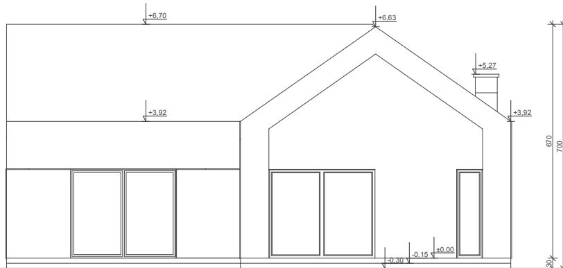
ELEWACJA OGRODOWA
