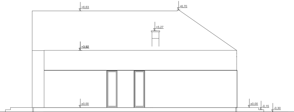
ELEWACJA BOK 1
