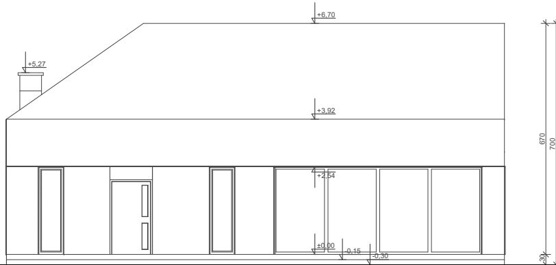
ELEWACJA FRONTOWA
